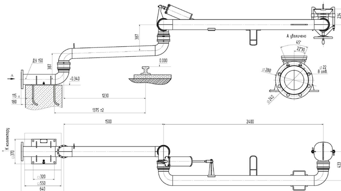
Рис. 4. Установочные и габаритные размеры стояка ОСН-СНС-150-6
